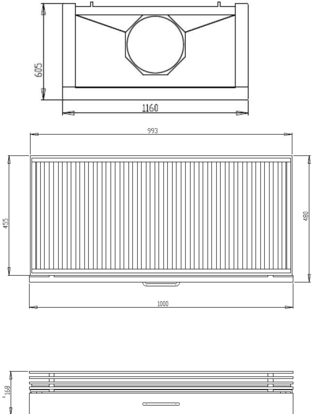
Stalen rookkap
