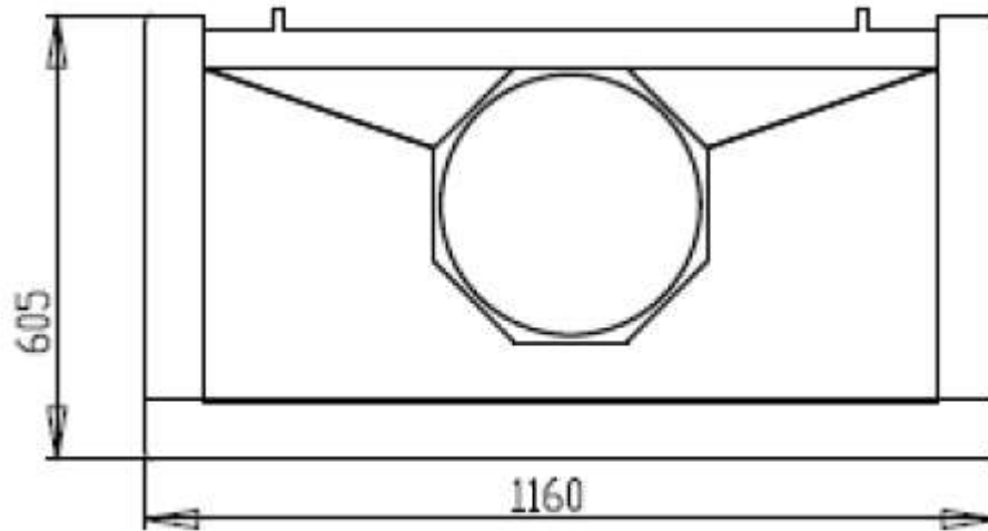
Stalen rookkap
